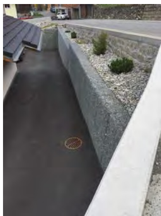
EINFACHE DRAHTGABIONEN
