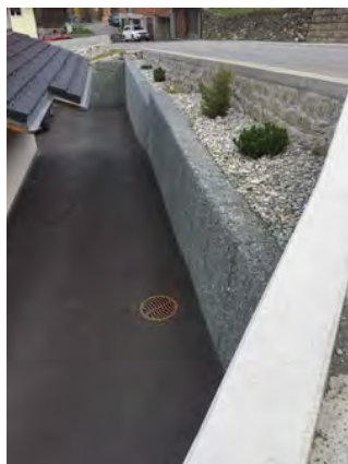
GABIONS SIMPLE FILS
